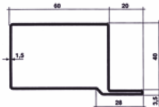
15B kg/m 2,72
