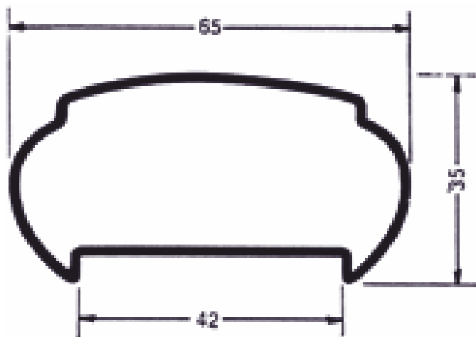
MT7 - 15/10=kg/ml 2,15
