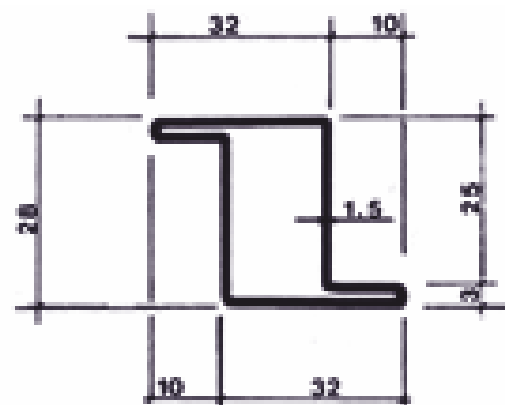
11C kg/m 1,57
