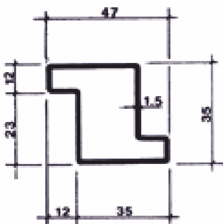
2Z kg/m 1,88
