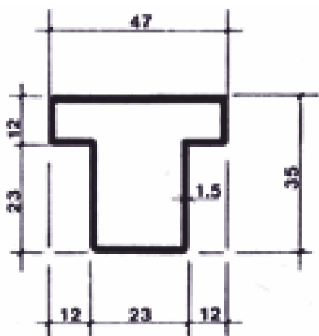
2B kg/m 1,88
