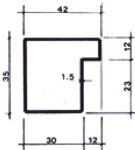
2A kg/m 1,76
