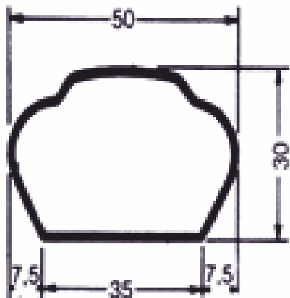
MT5 - 15/10=kg/ml 1,65
