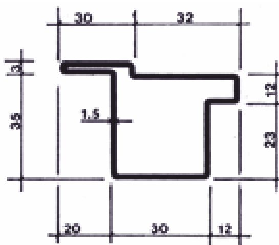
2T kg/m 2,30
