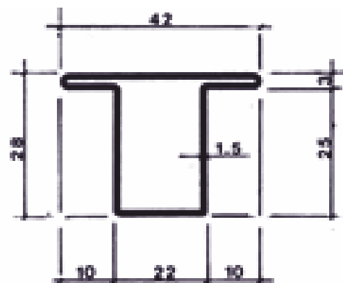
11B kg/m 1,57
