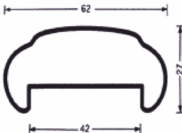
MT8 - 15/10=kg/ml 1,87
