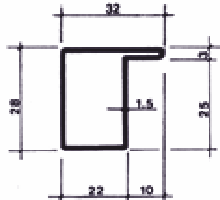
11A kg/m 1,34
