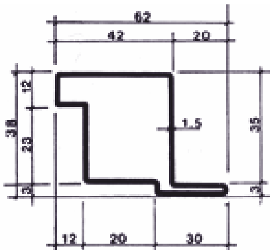
2N kg/m 2,30
