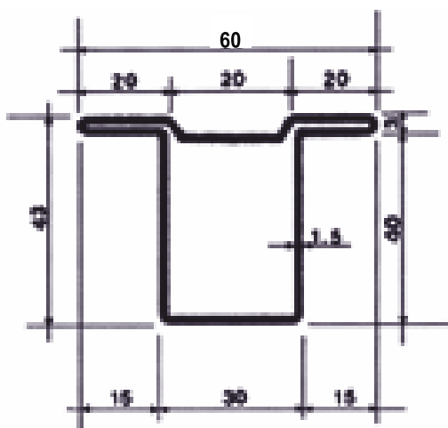
15T kg/m 2,45
